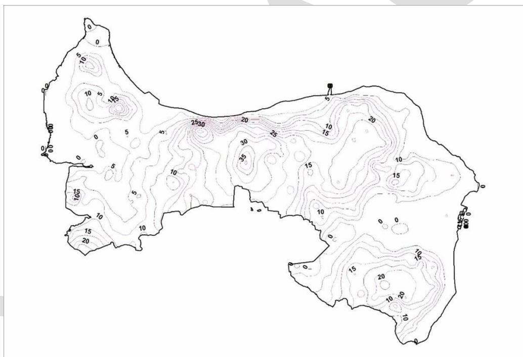
Figur 3.7 Kort over grundvandspotentialerforhold (Århus Amt 2006).
