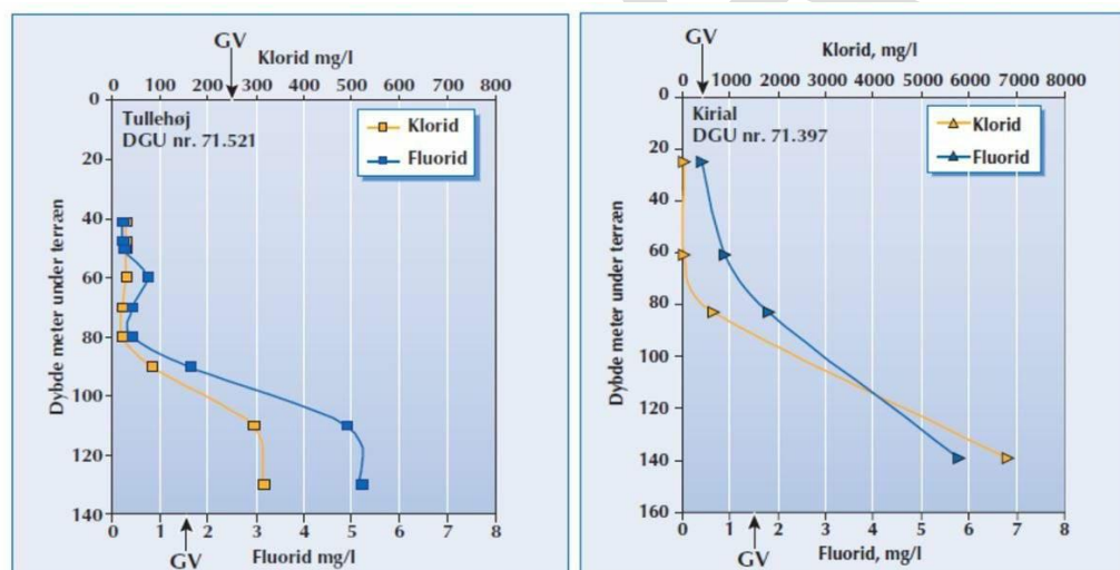
Figur 3.6 Klorid og fluorid som funktion af dybden i boringen DGU-nr. 71.521, som ligger nord for Skindbjerg og boringen DGU-nr. 71.397, som ligger ved Kirial. Der kan kun indvindes anvendeligt drikkevand i de øverste ca. 70 m under terræn. Det dybereliggende grundvand er uegnet pga. høje indhold af klorid og fluorid. (Århus Amt 2005)
