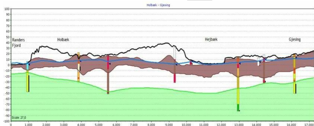
Figur 3.5 Geologisk tværsnit fra Holbæk til Gjesing
