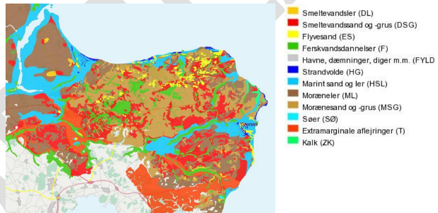
Figur 3.3 Jordartskort (GEUS)
